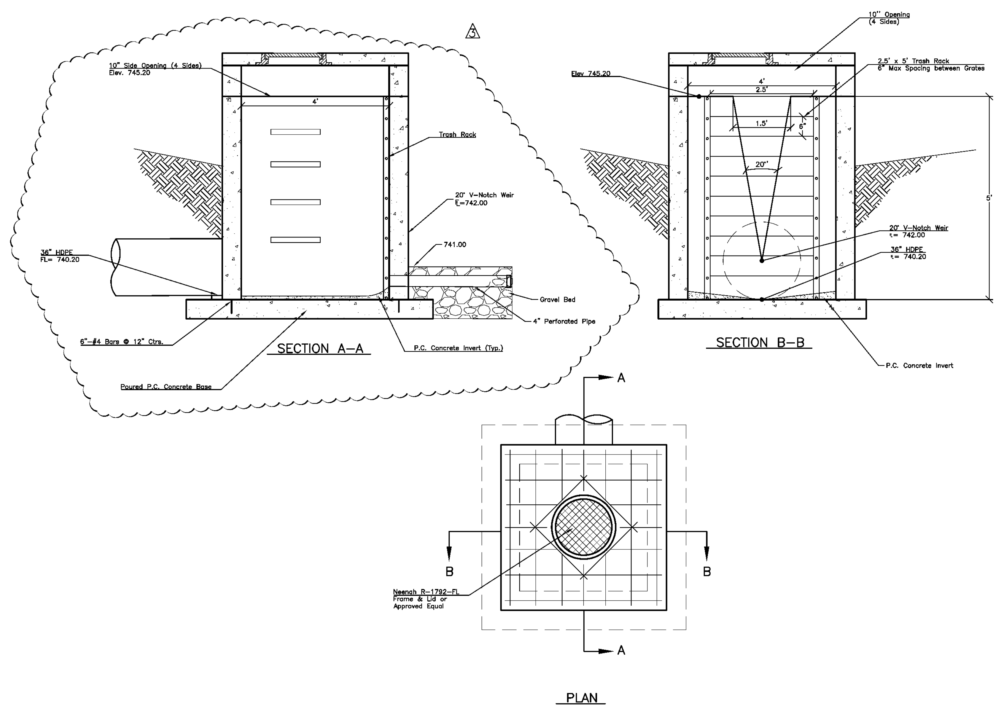
2 PRECAST DRY DETENTION BMP OUTLET STRUCTURE C0.35 N.T.S.
